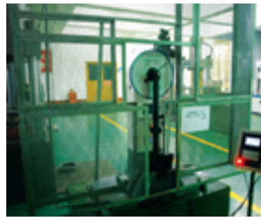
冲击试验机
